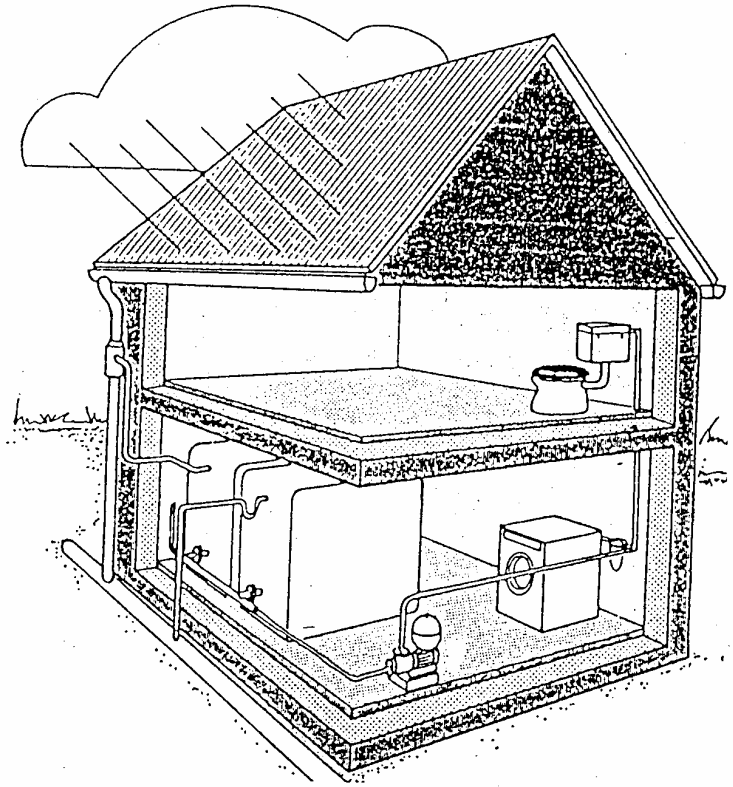
Beispiel für Anlage mit Innentanks und Fallrohr- filter.
